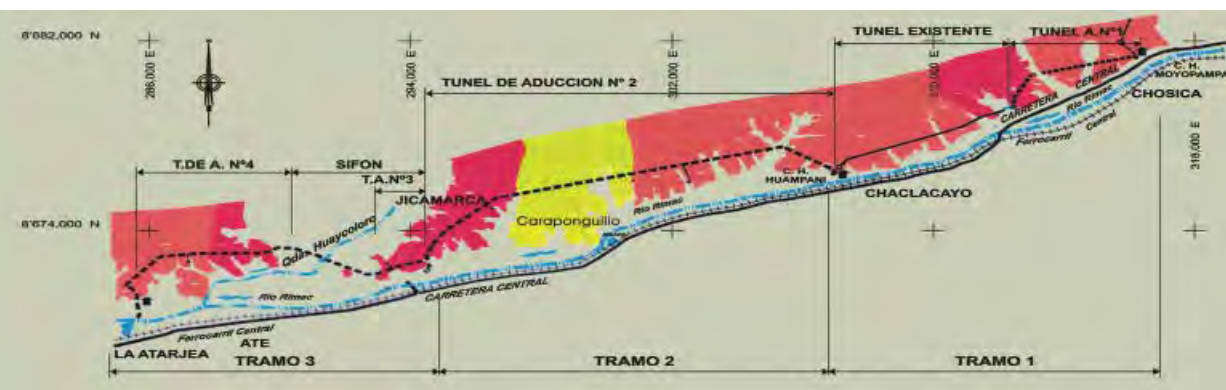
Conducción hidráulica fuera del cauce del río Rímac. Hydraulic diversion out of Rímac river bed.
